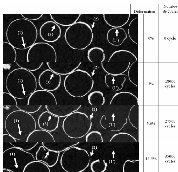
FIG. 4 – Visualisation des mécanismes d'endommagement en fatigue des empilements de sphères creuses en Ni+NiB observés sur des coupes obtenues par tomographie aux rayons X.
