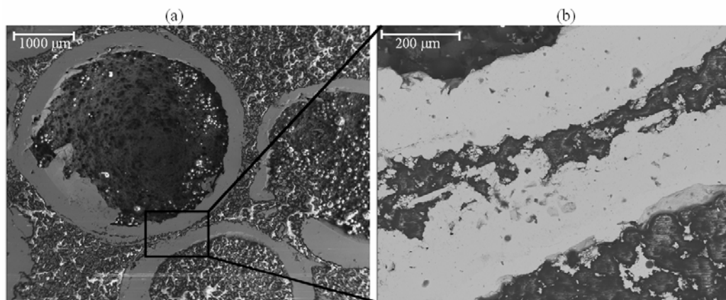
FIG. 1 – Images MEB d'un empilement de sphères creuses en Nickel + Nickel Bore (a) Aux électrons secondaires (x20) (b) Etude du col de liaison aux électrons rétrodiffusés grossissement (x120).
