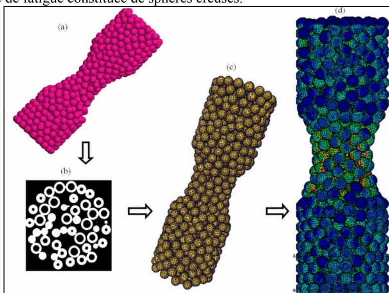
FIG. 5 – Résumé des étapes de construction d'un calcul EF à partir d'images d'empilements générées numériquement (a) Visualisation de l'empilement gravitaire numérique. (b) Coupe de l'empilement lié. (c) Maillage EF réalisé à partir de l'image (d) Calcul EF en élasticité linéaire (Abaqus standard), observation des isocontraintes de Von Mises.
