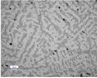
Figure (5) : Observation micrographique de l'échantillon A
