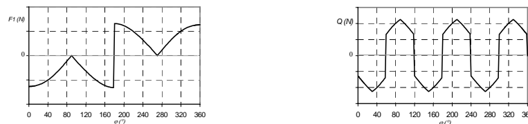
FIG 7 – Allure de l'effort axial généré par 1 (à gauche) ou les 3 galets (à droite) sur un tour
