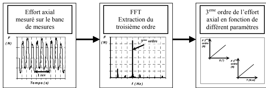
FIG 3 – Post-traitement des mesures effectuées sur le banc
