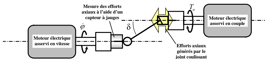
FIG 2 – Schéma de principe du banc de mesure
