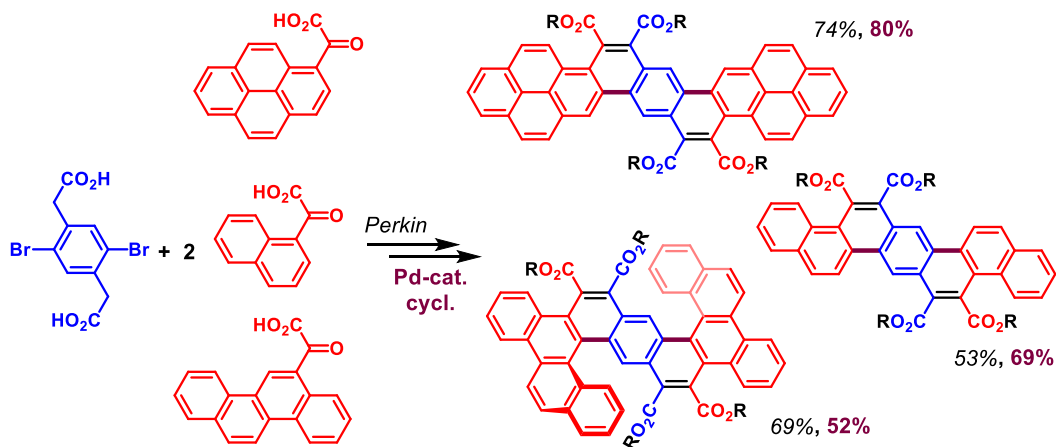
Figure 3 : Courts rubans aromatiques obtenus par réaction de Perkin suivie de déshydrobromation.
