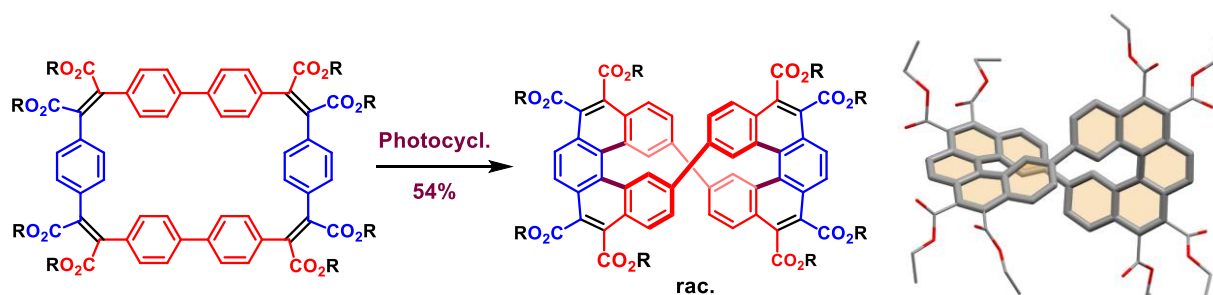
Figure 9 : Synthèse et structure du cyclo-bis-[5]héliène.
