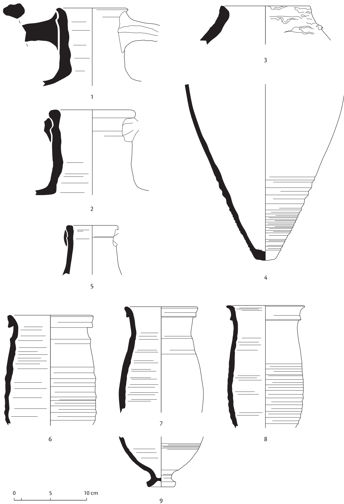
FIG. 2. Mobilier amphorique et pots de saqia provenant des niveaux de remblais recouvrant les salles chaudes du complexe (MFFTP/J. Marchand).
