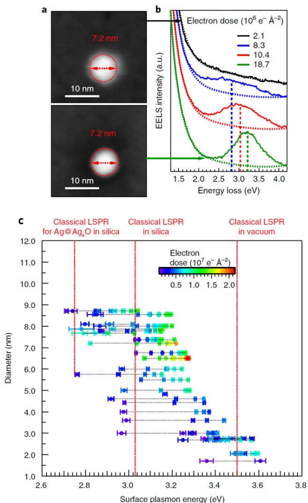
Figure 5. (a) Evolución de los espectros EELS de una nanoesfera de plata con la dosis de electrones. (b) Evolución de la posición del pico del plasmón de superficie dipolar con el tamaño de las nanopartículas de plata y con la dosis de electrones. Tomado de [20].
