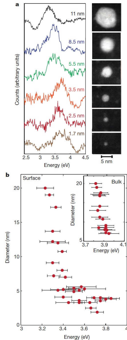
Figure 2. (a) Espectros EELS de nanoesferas de plata de diferentes tamaños. Las imágenes de las nanopartículas corresponden a imágenes obtenidas por un microscopio de tipo STEM. (b) Evolución de la posición del pico del plasmón de superficie dipolar con el tamaño de las nanopartículas de plata. Arriba a la derecha también aparece la evolución de la señal EELS proveniente del interior (bulk) de las partículas. Tomado de [25].
