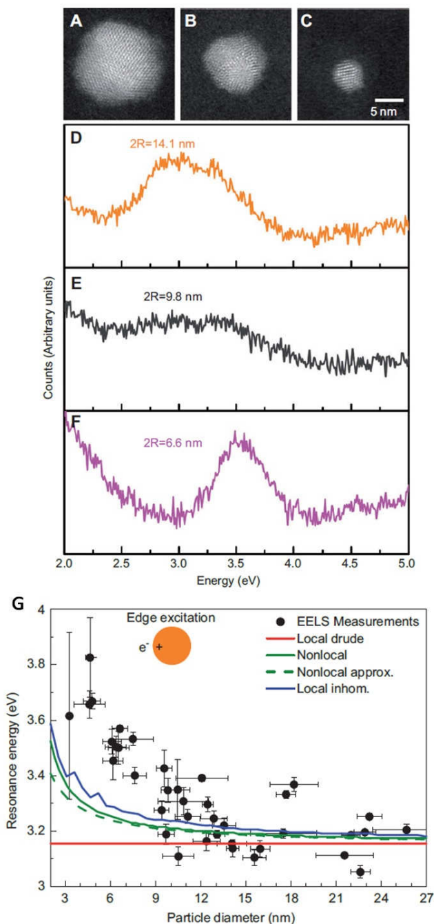
Figure 3. (a-c) Imágenes de microscopía STEM de diferentes tamaños de nanopartículas de plata. (d-f) Evolución de los espectros EELS de nanoesferas de plata de tamaño decreciente. g) Evolución de la posición del pasmón de superficie dipolar con el tamaño de nanopartícula de plata (puntos negros). En rojo, verde, verde punteado y azul vemos diferentes modelos teóricos. Tomado de [26].
