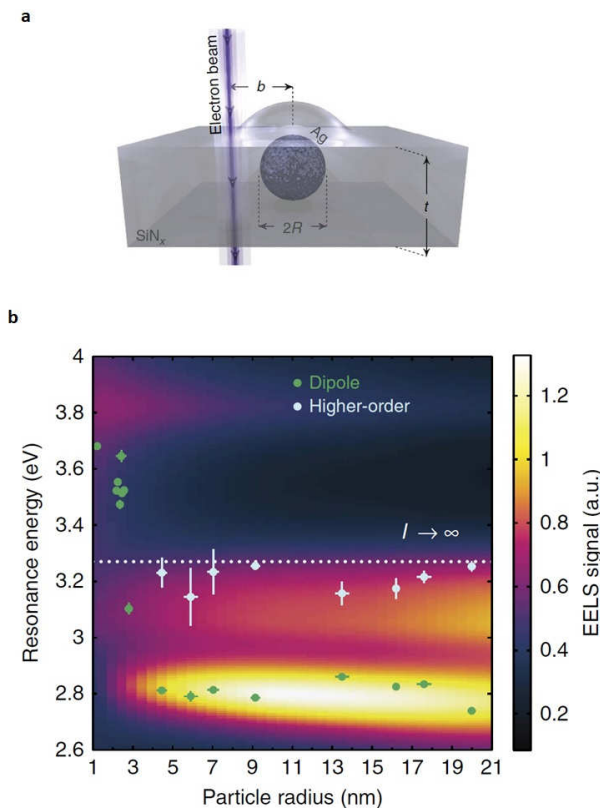
Figure 4. (a) Sistema de nanopartícula de plata dentro de un medio homogéneo de \text{SiN}_x estudiado por la técnica EELS en la referencia [27]. (b) Evolución de la energía del plasmón de superficie dipolar (en puntos verdes) con el tamaño de las nanopartículas. El fondo amarillo en la gráfica representa los resultados predichos por simulaciones EELS clásicas.
