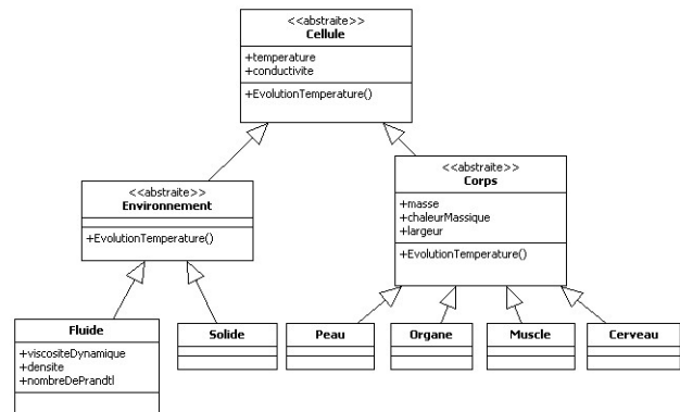
Figure 2: Classes des cellules de l'automate
