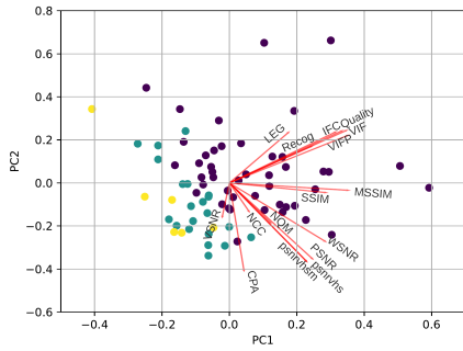
(a) H.265
