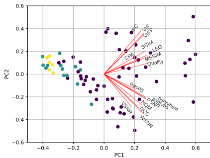
(d) jxr
