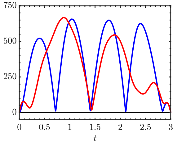
Figure 5: c_g = 10 – Evolution of \|v_4(\cdot, t)\|_{L^2_\chi(\omega)} (—), and \|v_0(\cdot, t)\|_{L^2_\chi(\omega)} (—) w.r.t. t .
