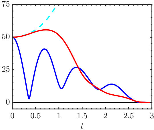
Figure 6: c_f = 10 - \|v_4(\cdot, t)\|_{L^2_\chi(\omega)} (—), and \|v_0(\cdot, t)\|_{L^2_\chi(\omega)} (—) w.r.t. t .
