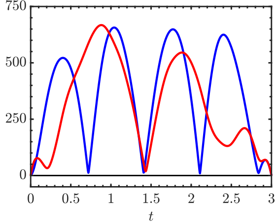
Figure 6: c_f = 10 - \|v_4(\cdot, t)\|_{L^2_\chi(\omega)} (—), and \|v_0(\cdot, t)\|_{L^2_\chi(\omega)} (—) w.r.t. t .
