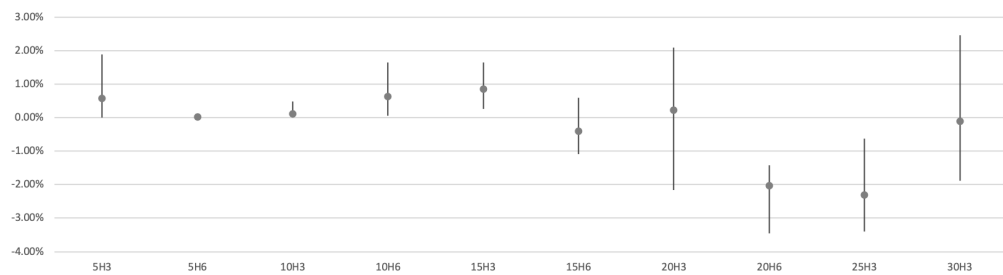
(d) |\mathcal{M}| = 120
