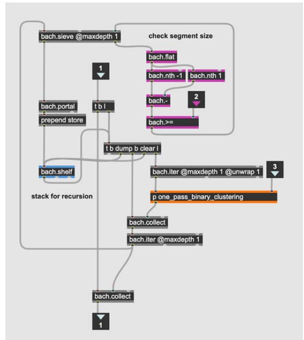
Figure 12. Implémentation en MAX/MSP et librairie bach de l'algorithme de clustering récursif. L'objet one_pass_binary_clustering correspond au code de fig. 11.
