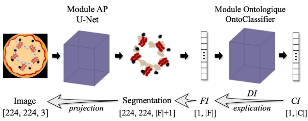
FIGURE 4 – Classifieur ontologiquement explicable.
