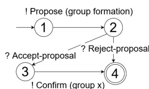
FIGURE 2 – Protocole de proposition de formation de groupe
