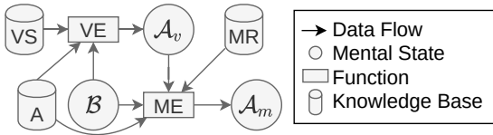
FIGURE 3 – Architecture des agents juges, adaptée d’Ethicaa [13].
