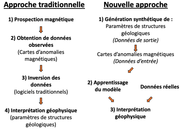
FIGURE 2 – Schéma de la dynamique traditionnelle suivie en géophysique (à gauche), et celui de la nouvelle approche proposée dans cette étude (à droite).
