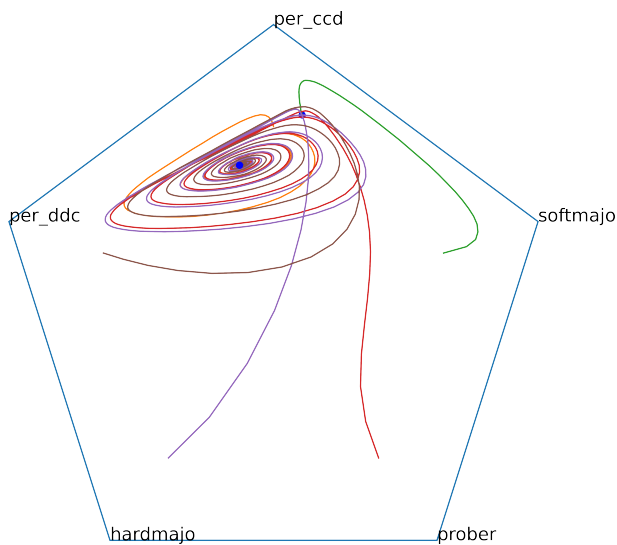
FIGURE 5 – À partir des mêmes stratégies que la figure précédente, représentation barycentrique avec un calcul utilisant des entiers. Avec des réels, l’image est quasiment identique.
