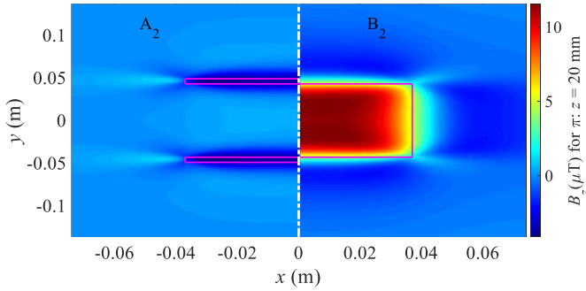
Fig. 8. Composantes z des résultats du champ magnétique produit par la boucle de courant de sortie d'un PCA _{4 \times 3} sur un plan parallèle au plan des interconnexions à z = 20 mm en considérant le trajet de retour A (gauche) ; et le trajet de retour B (droite). Grâce aux symétries, seules les demi-boucles sont tracées.
