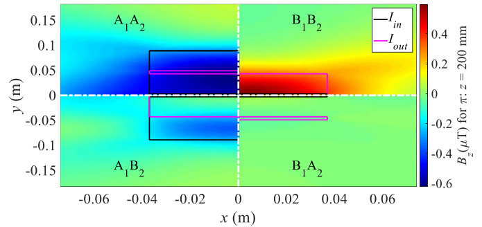
Fig. 11. Résultats des composantes z du champ magnétique produit par les 4 combinaisons de boucles d'un PCA _{4 \times 3} sur un plan parallèle au plan des interconnexions à z = 200 mm. Grâce aux symétries, seules les 1/4 boucles sont tracées.
