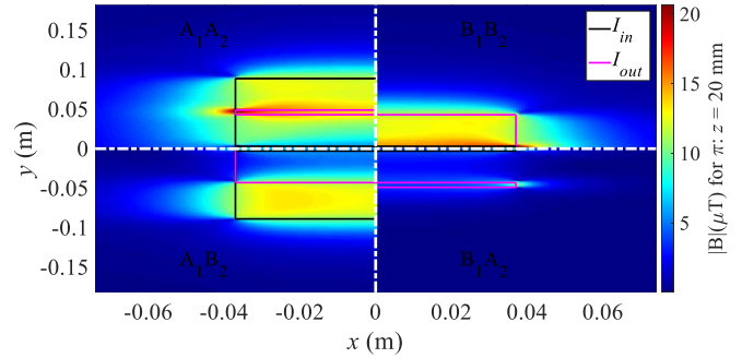
Fig. 10. Résultats des composantes z du champ magnétique produit par les 4 combinaisons de boucles d'un PCA _{4 \times 3} sur un plan parallèle au plan des interconnexions à z = 200 mm. Grâce aux symétries, seules les boucles 1/4 sont tracées.
