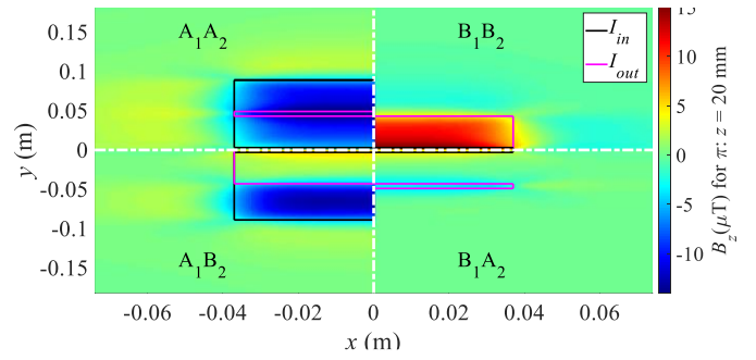
Fig. 9. Résultats des composantes z du champ magnétique produit par les 4 combinaisons de boucles d'un PCA _{4 \times 3} sur un plan parallèle au plan des interconnexions à z = 20 mm. Grâce aux symétries, seules les 1/4 boucles sont tracées.
