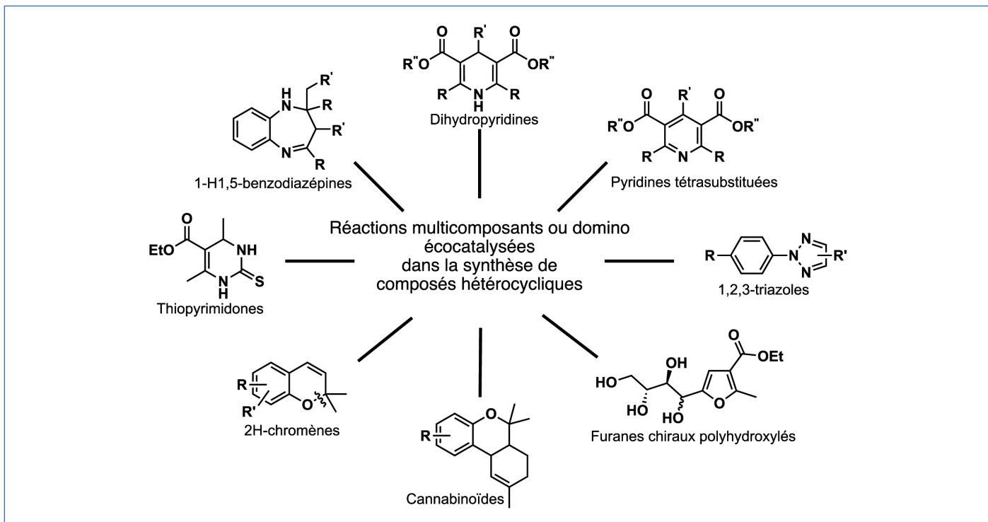
Figure 6 - Synthèses écocatalysées d'hétérocycles.
