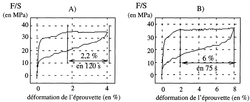
Figure 3. Réponses mécaniques de l'éprouvette pour deux valeurs du coefficient d'échange thermique ( h_A < h_B ).
