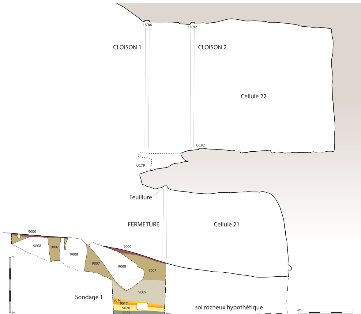
Fig. 11. Coupe des cellules 21 et 22. Coupe ouest du sondage 1 (M. Liboutet).
