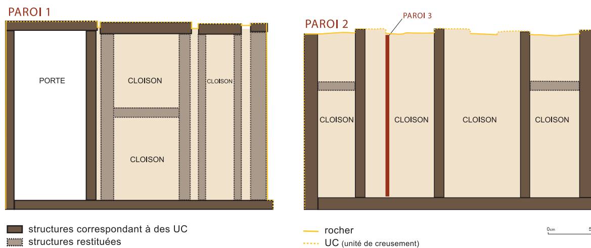
Fig. 13. Restitution des cloisons 1 et 2 en pans de bois de la cellule 20 (D. Glauser, M. Liboutet).
