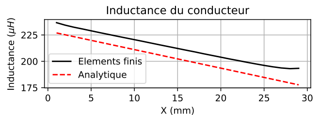
Figure 9. Comparaison des inductances pour N_s = 20 spires obtenues de manière «Analytique» (5) et par le modèle «Éléments finis».
