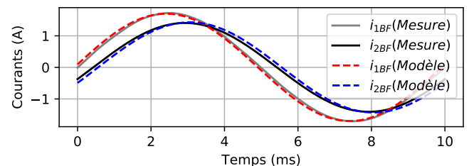
Figure 12. Composantes fondamentales des courants mesurés (Figure 10) et simulés (10) sous une consigne de courant de 2A à 100Hz (enroulement 1 maître/ enroulement 2 esclave).
