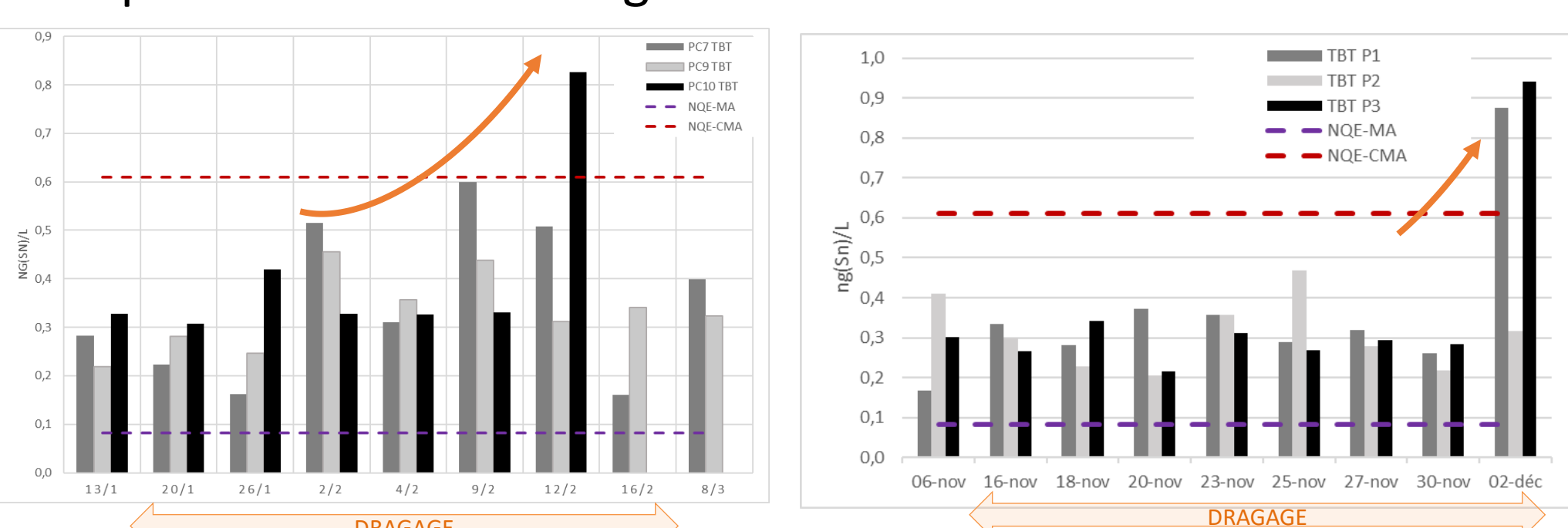
Figure 3 : Concentrations en TBT mesurées au cours des dragages de Port-Camargue et Pérols
