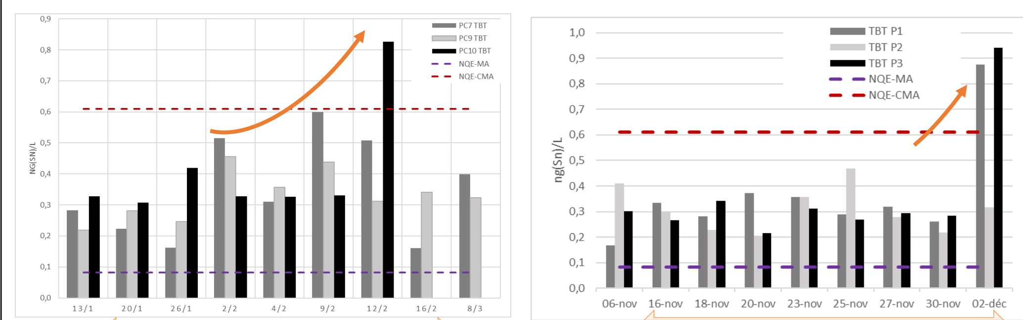
Figure 3 : Concentrations en TBT mesurées au cours des dragages de Port-Camargue et Pérols
