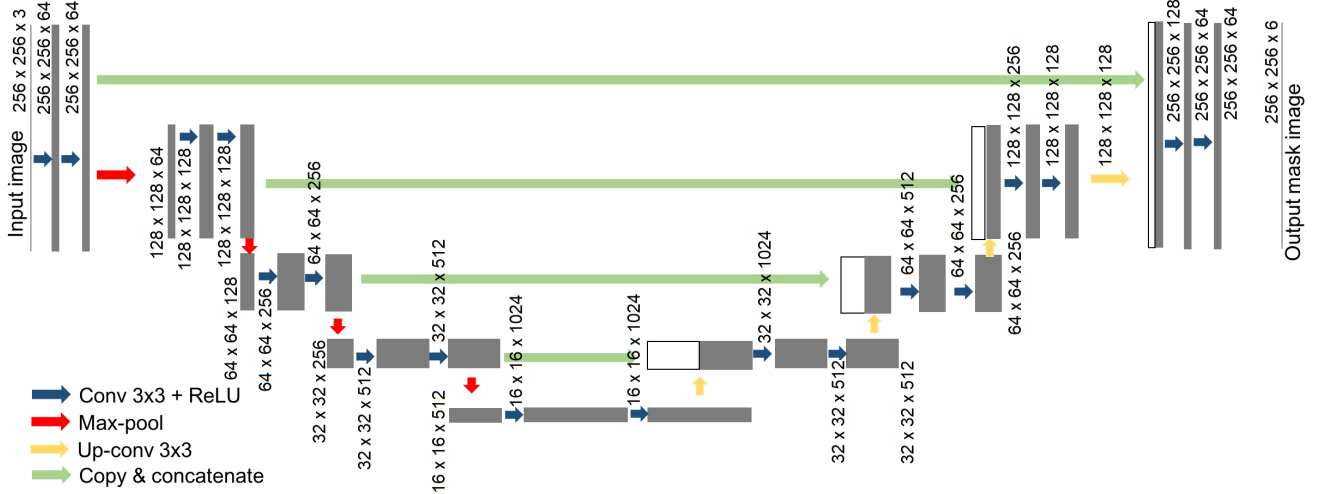
FIGURE 2 – Architecture d’un réseau U-Net [6].
