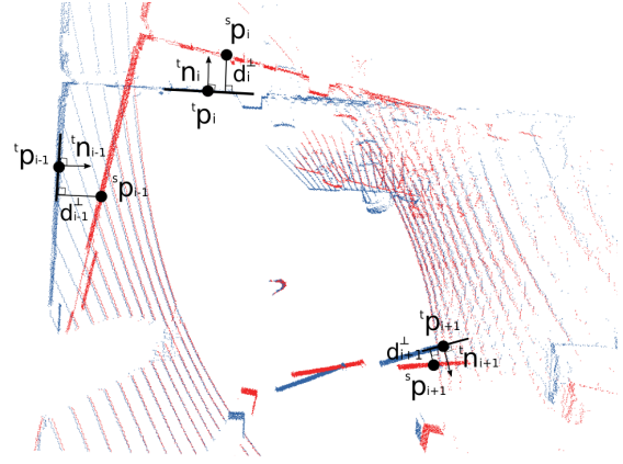
FIGURE 3 – Distance point à plan d_i^\perp comme décrit dans [3]. En bleu, le nuage de points cible et les normales de surface liées à ses points. En rouge, le nuage de points source à recalquer.
