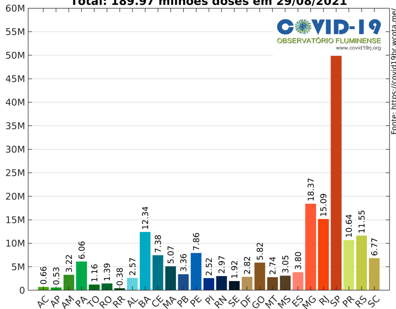
Doses de vacinas contra COVID-19 aplicadas no Brasil (em milhões) Total: 189.97 milhões doses em 29/08/2021
