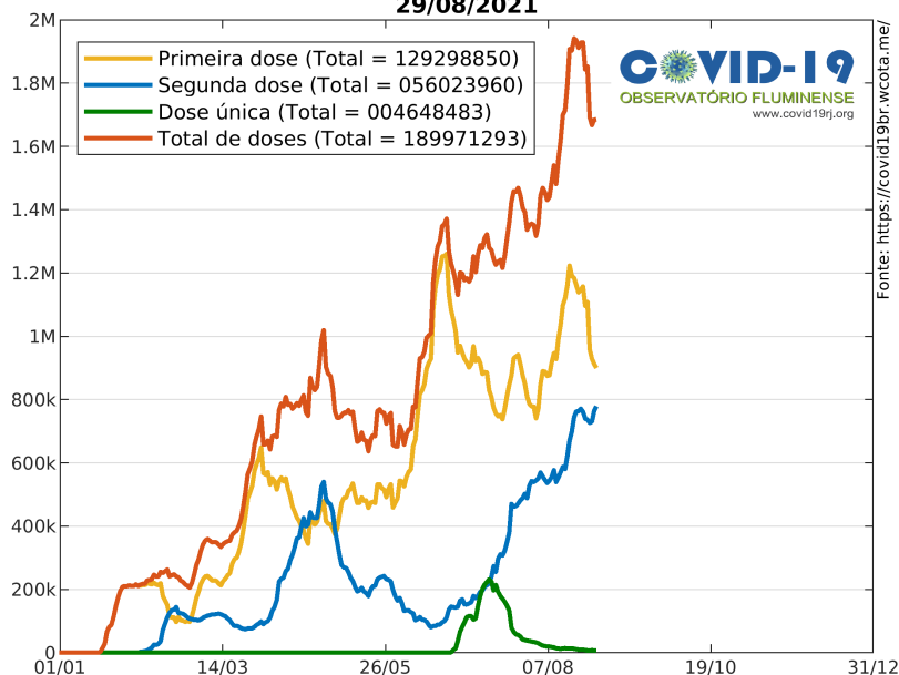
Média móvel de 7 dias da vacinação diária contra COVID-19 no Brasil 29/08/2021
