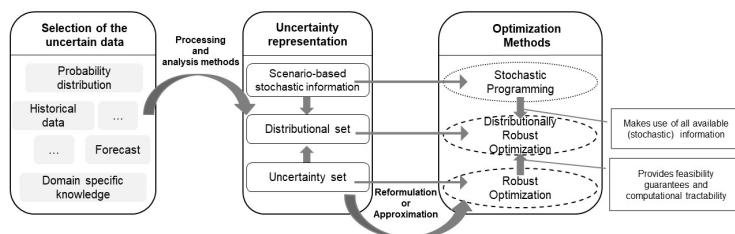
Fig. 1. DDO framework
