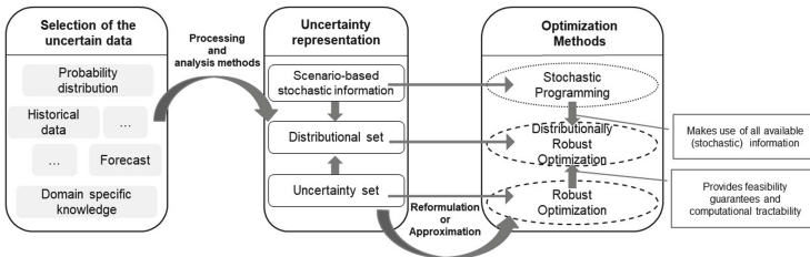
Fig. 1. DDO framework
