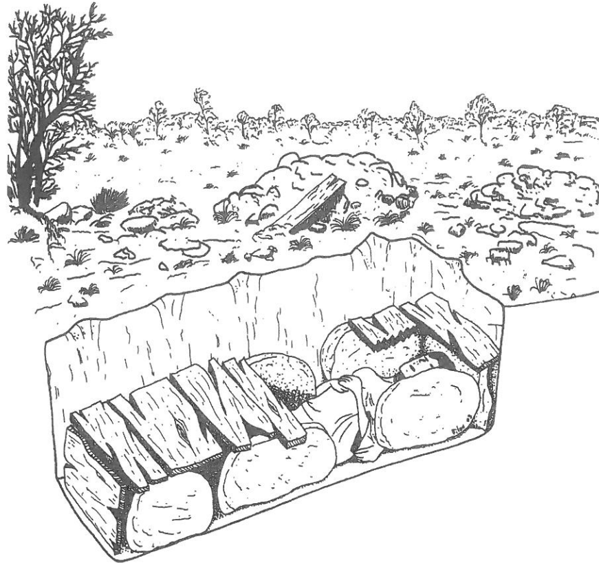
Fig. 8 – Restitution d'un coffrage mixte (dessin Philippe Blanchard).
