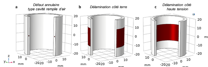
Fig. 8. Représentation en 3D d'un isolateur solide cylindrique contenant trois types de discontinuités localisées (défauts remplis d'air, en rouge).
