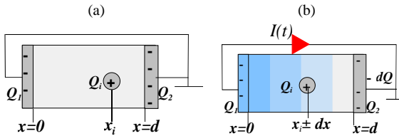
Fig. 4. Principe de la méthode de l'onde thermique (exemple pour un échantillon plan en court-circuit). (a) : La présence d'une charge d'espace Q_i dans l'échantillon induit des charges d'influence Q_1 et Q_2 aux électrodes. (b) : Lorsque l'équilibre électrostatique de l'échantillon est perturbé par la diffusion de la température dans le matériau (dilatation/contraction, variations locales de la permittivité avec la température), des variations des charges d'influence aux électrodes ( Q_2-dQ et Q_1+dQ , respectivement) ont lieu pour le rétablir. Le transport de charge dQ d'une électrode à l'autre à travers le circuit extérieur donne ainsi naissance à une réponse transitoire en courant I(t) = -dQ/dt .
