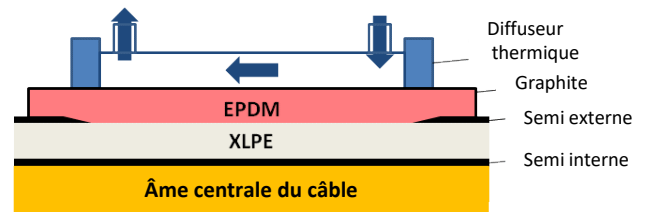
Fig. 5. Représentation axisymétrique de la configuration bi-couche étudiée, comportant l'isolation du câble (XLPE) et la couche en EPDM représentant le matériau utilisé dans une jonction HVDC [14].
