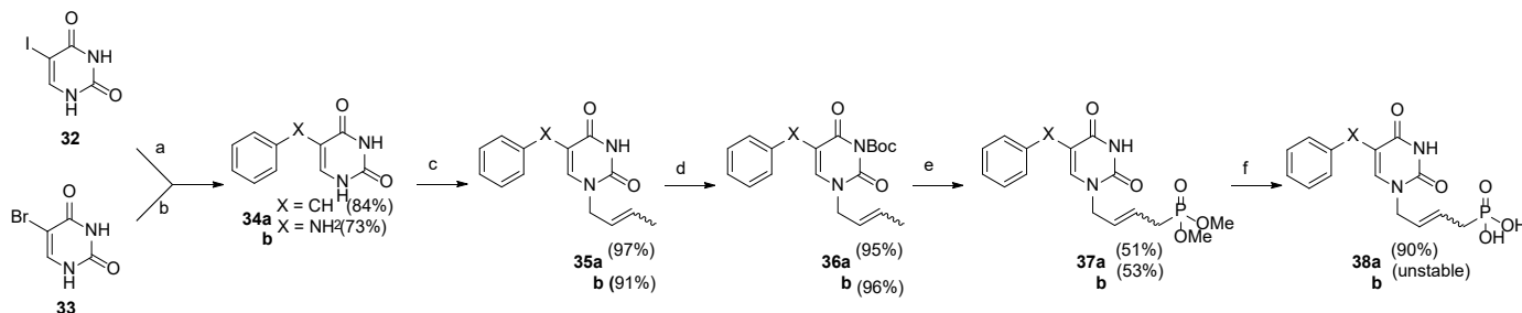
Scheme 5: reagents and conditions: (a) for ( 34a ): i) MeMgCl.LiCl, -20 °C, 30 min, THF, ii) iPrMgCl.LiCl, -20 °C, 30 min, 2h, rt. iii) CuI 2 .LiCl, -30 °C to rt, 1 h, iv) BnBr, rt, 12 h.; (b) for ( 34b ): aniline, 175 °C, 20 min.; (c) i) BSA, CH 3 CN, MW, 5 min, 80 °C, ii) TMSCl, crotyl bromide, Na 1 act, MW, 30 min, 80 °C; (d) Boc 2 O, DMAP, THF, MW, 10 min. 70 °C; (e) i) allylphosphonate, G-II, DCM Anh , ii) 80 kHz, 55 °C, 24 h, ii) TFA, DCM, rt, 6 h.; (f) TMSBr, ACN Anh , MW, 70 °C, 10 min.
