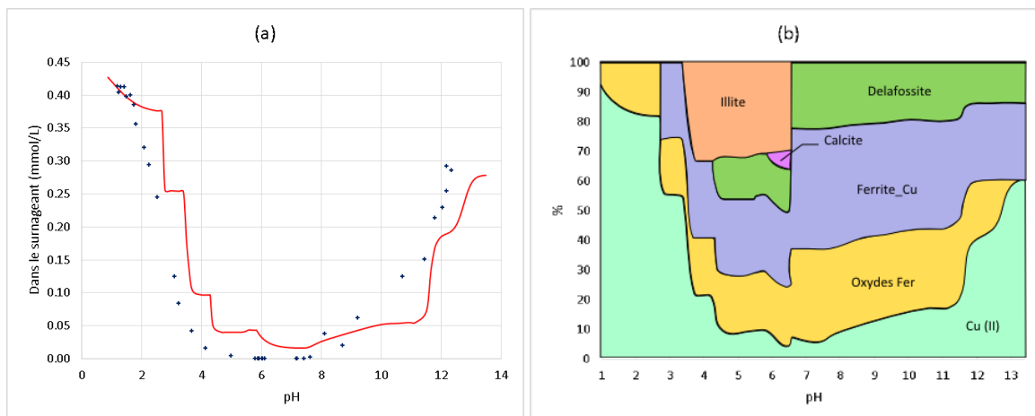
Figure 2 : Relargage du cuivre en fonction du pH (a), spéciation du cuivre en fonction du pH (b), Expérimental : croix, modélisation : ligne
