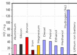
Densité énergétique par kilogramme de carburant [1]
