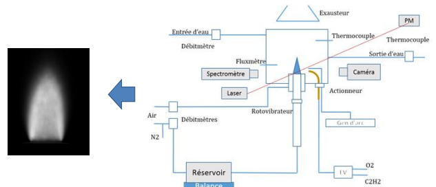
Schéma expérimental du brûleur mis en place et flamme d'aluminium stabilisée
