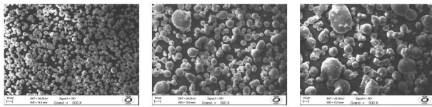
Visualisation par MEB d'un ensemble de particules d'aluminium.
