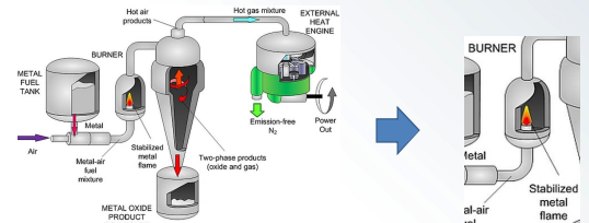
Illustration d'un convertisseur énergétique [2].
