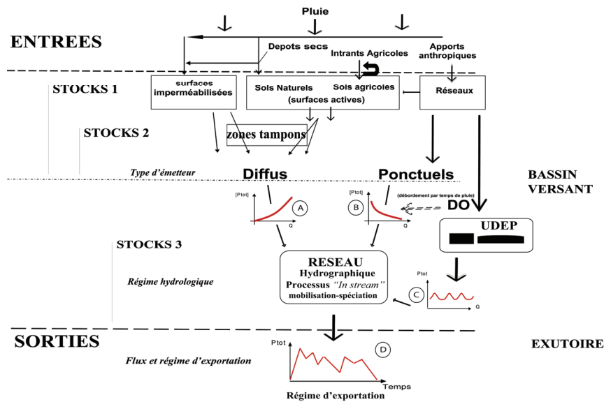
Figure 1 : Représentation d'un système de transfert du P dans un bassin versant péri-urbain d'après Dorioz et Poulénard (2007) modifiée. (P tot) = concentration en phosphore total. (Q)=débit, UDEP= usine de dépollution des eaux usées. Les entrées aux systèmes sont potentiellement transmises au réseau hydrographique ou stockées puis fixées ou remobilisées. Le dernier stock est le réseau hydrographique lui même où peut s'opérer une spéciation du P. La courbe A décrit le comportement de concentration des flux, issu des émetteurs du diffus, corrélé à l'augmentation du débit. La courbe B décrit le comportement de dilution par l'augmentation du débit, des apports des émetteurs ponctuels, la courbe C décrit la cyclicité des rejets de station de traitement en fonction du temps, à débit sensiblement égal, enfin la courbe D décrit la variabilité des concentration de Ptot à l'exutoire en fonction du temps. Le jeu de ces systèmes de transferts détermine à l'exutoire, la nature, l'intensité et le régime d'exportation des flux.
