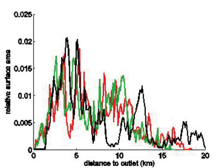
Figure 5: Comparaison de la distribution des distances à l'exutoire pour les trois estimations de réseau de drainage sur le bassin de la Chézine (approche MNT en vert, approche objet en rouge et approche TIN en noir)
