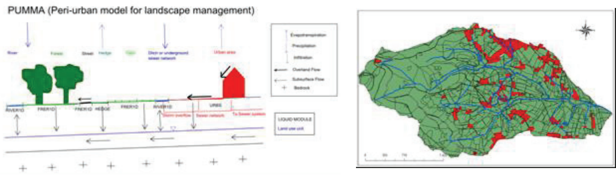
Figure 7: (a) Schéma du modèle PUMMA et des flux entre les différents objets. (b) Discrétisation spatiale du bassin du Mercier pour la modélisation. En rouge : les parcelles urbaines où on applique le module UBRS. En vert : les parcelles naturelles où on applique le module FRER1D et en bleu : le réseau naturel + fossés où on applique le module RIVER1D.
