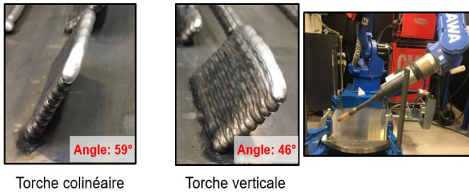
Figure 7. FABRICATION DE DEUX MURS INCLINES AVEC DEUX STRATEGIES DIFFERENTES
