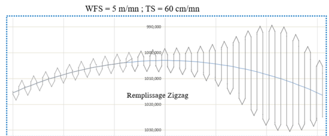
Figure 12. STRATEGIE DE REMPLISSAGE EN ZIGZAG
