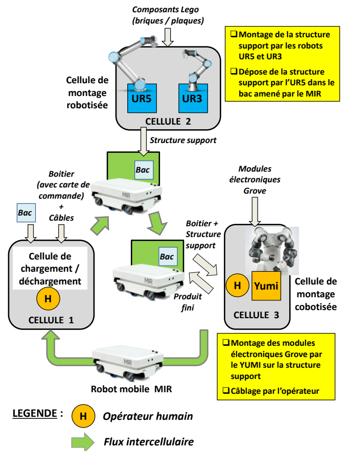
Figure 5. DESCRIPTION DU PROCESSUS DE MONTAGE
