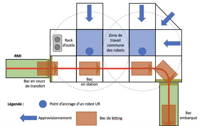
Figure 3. EXEMPLE D'AGENCEMENT D'UNE CELLULE AVEC SES MOYENS LOGISTIQUES INTRA ET INTER CELLULAIRES
