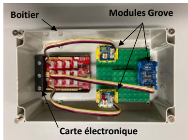
Figure 4. ELEMENTS CONSTITUTIFS DU PRODUIT
