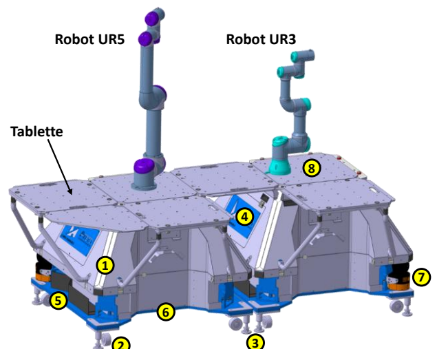
Figure 2. ASPECT MATERIEL D'UNE CELLULE AVEC DEUX UEC
