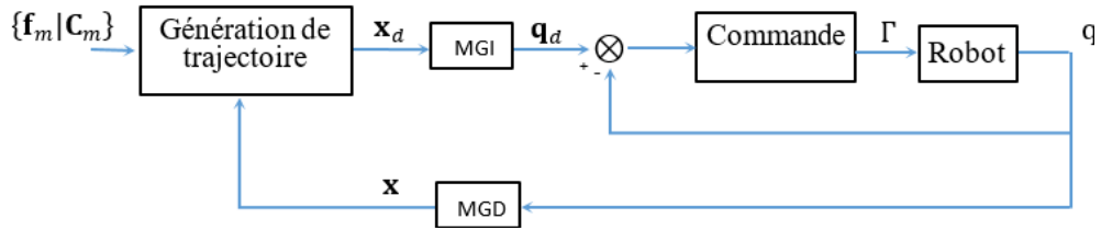
Figure 7. SCHEMA CLASSIQUE DE GENERATION DE MOUVEMENT DANS L'ESPACE OPERATIONNEL
