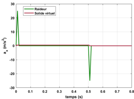
Figure 11. COURBES D'ACCELERATIONS A_x DE L'EFFECTEUR SUIVANT LA DIRECTION DE L'EFFORT APPLIQUE
