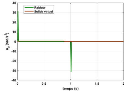
Figure 13. COURBES DE VITESSE ANGULAIRE V_\theta ET ACCELERATION ANGULAIRE A_\theta DU REPERE LIE A L'EFFECTEUR SELON LA DIRECTION DU COUPLE APPLIQUE, AVEC UN GENERATEUR DE TRAJECTOIRE DE TYPE SOLIDE VIRTUEL ET RAIDEUR.
