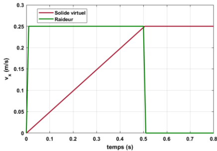
Figure 10. COURBES DE VITESSES V_x SUIVANT LA DIRECTION DE L'EFFORT APPLIQUE
