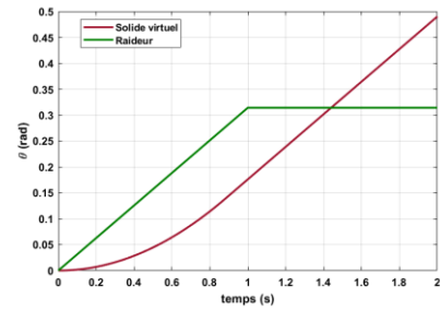
Figure 12. COURBES DE POSITION ANGULAIRE \theta GENEREES PAR LA METHODE DU SOLIDE VIRTUEL ET PAR LA METHODE EN RAIDEUR SUIVANT LA DIRECTION DU COUPLE APPLIQUE
