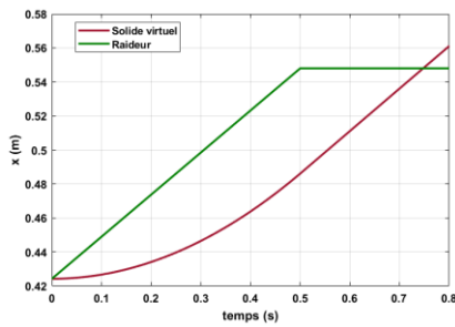
Figure 9. POSITIONS CARTESIENNES X GENEREES PAR LA METHODE DU SOLIDE VIRTUEL ET PAR LA METHODE EN RAIDEUR SUIVANT LA DIRECTION DE L'EFFORT APPLIQUE
