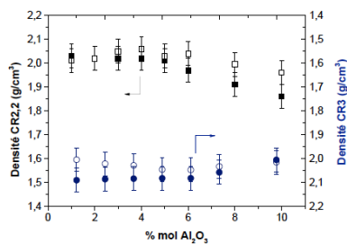
Figure IV-10 : Densités calculées (marqueurs vides) et expérimentales (marqueurs pleins) [5] en fonction du % molaire d'alumine dans le système \text{NaF-AlF}_3\text{-Al}_2\text{O}_3 dans le liquide avec un CR ( \text{NaF}/\text{AlF}_3 ) de 2,2 (symboles carrés) et CR 3 (symboles cercles).
