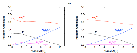
Figure IV-8 : Fractions anioniques déduites des déplacements chimiques de la RMN à haute température pour les systèmes fondus \text{MF-AlF}_3\text{-Al}_2\text{O}_3 ( \text{M} = \text{Na} à gauche et \text{M} = \text{K} à droite) pour un CR 2,2.
