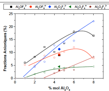
Figure V-11 : Fractions anioniques des oxyfluoroaluminates en fonction de l'alumine pour le système fondu NaF-AlF 3 -Al 2 O 3 à CR2,2 (lignes avec marqueurs vides) et le système avec 5 % massique de CaF 2 (en marqueurs pleins).
