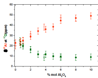
Figure IV-6 : Déplacements chimiques à haute température pour les noyaux ^{27}\text{Al} et ^{17}\text{O} du système \text{NaF-AlF}_3\text{-Al}_2\text{O}_3 avec un CR 2,2 (marqueurs pleins) et CR 3 (marqueurs vides).
