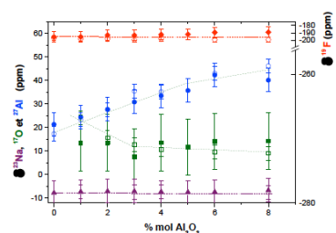
Figure IV-13 : Déplacements chimiques RMN dans le liquide des noyaux ^{27}\text{Al} (●○), ^{17}\text{O} (■□), ^{23}\text{Na} (▲△) dans l'axe principal et ^{19}\text{F} (◆◇) dans l'axe secondaire. Valeurs expérimentales en marqueurs vides et valeurs calculées en marqueurs pleins pour le système [\text{NaF}-\text{AlF}_3]_{\text{CR}3}-\text{Al}_2\text{O}_3 .
