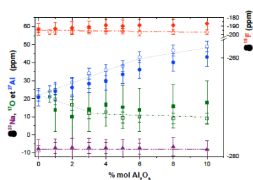
Figure IV-12 : Déplacements chimiques RMN dans le liquide des noyaux ^{27}\text{Al} (●○), ^{17}\text{O} (■□), ^{23}\text{Na} (▲△) dans l'axe principal et ^{19}\text{F} (◆◇) dans l'axe secondaire. Valeurs expérimentales en marqueurs vides et valeurs calculées en marqueurs pleins pour le système [\text{NaF}-\text{AlF}_3]_{\text{CR}2,2}-\text{Al}_2\text{O}_3 .
