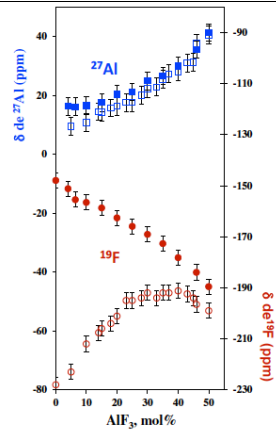
Figure III-3 : Déplacements chimiques à surchauffe constante de 20°C entre 0 à 50 % mol d' \text{AlF}_3 dans le système NaF-AlF 3 (symboles vides) et KF-AlF 3 (symboles pleins).
