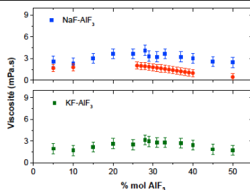
Figure III-33 : Viscosité des bains fondus MF-AlF 3 (M=Na, K) calculée à partir de la dynamique moléculaire à 1305 K (■ pour Na et ■ pour K). En rouge les données expérimentales [5], [151], [167] pour le système NaF-AlF 3 (panneau supérieur de la figure).
