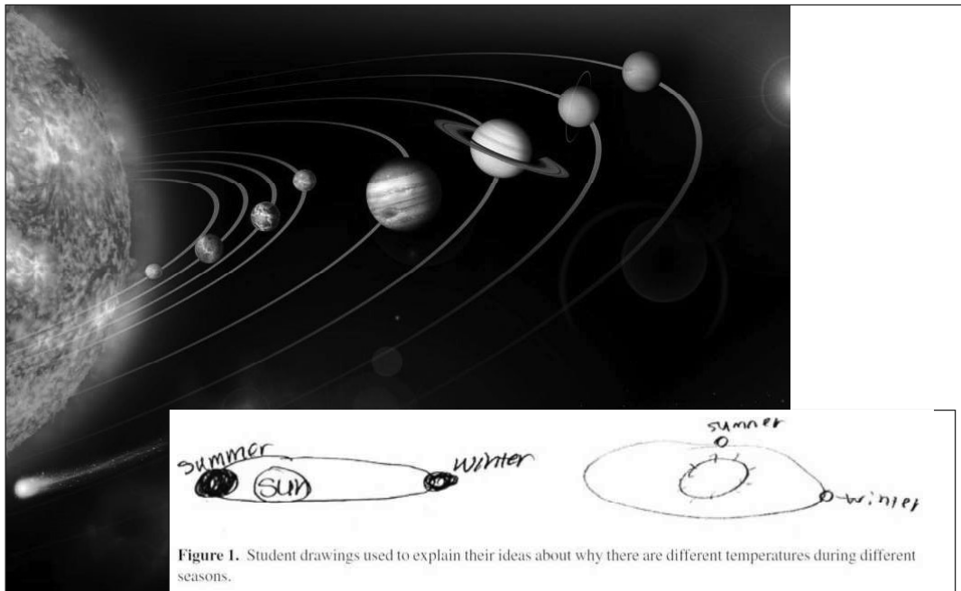
Figure 3. Les orbites planétaires sont souvent représentées comme des ellipses sur les sites Internet (gauche, futura-sciences.com © NASA) ou les manuels qui peuvent conduire à des représentations erronées sur les saisons (à droite, Lee, 2010, page 2). La représentation correcte est donnée par exemple sur le site de Pierre Causeret (2015).
