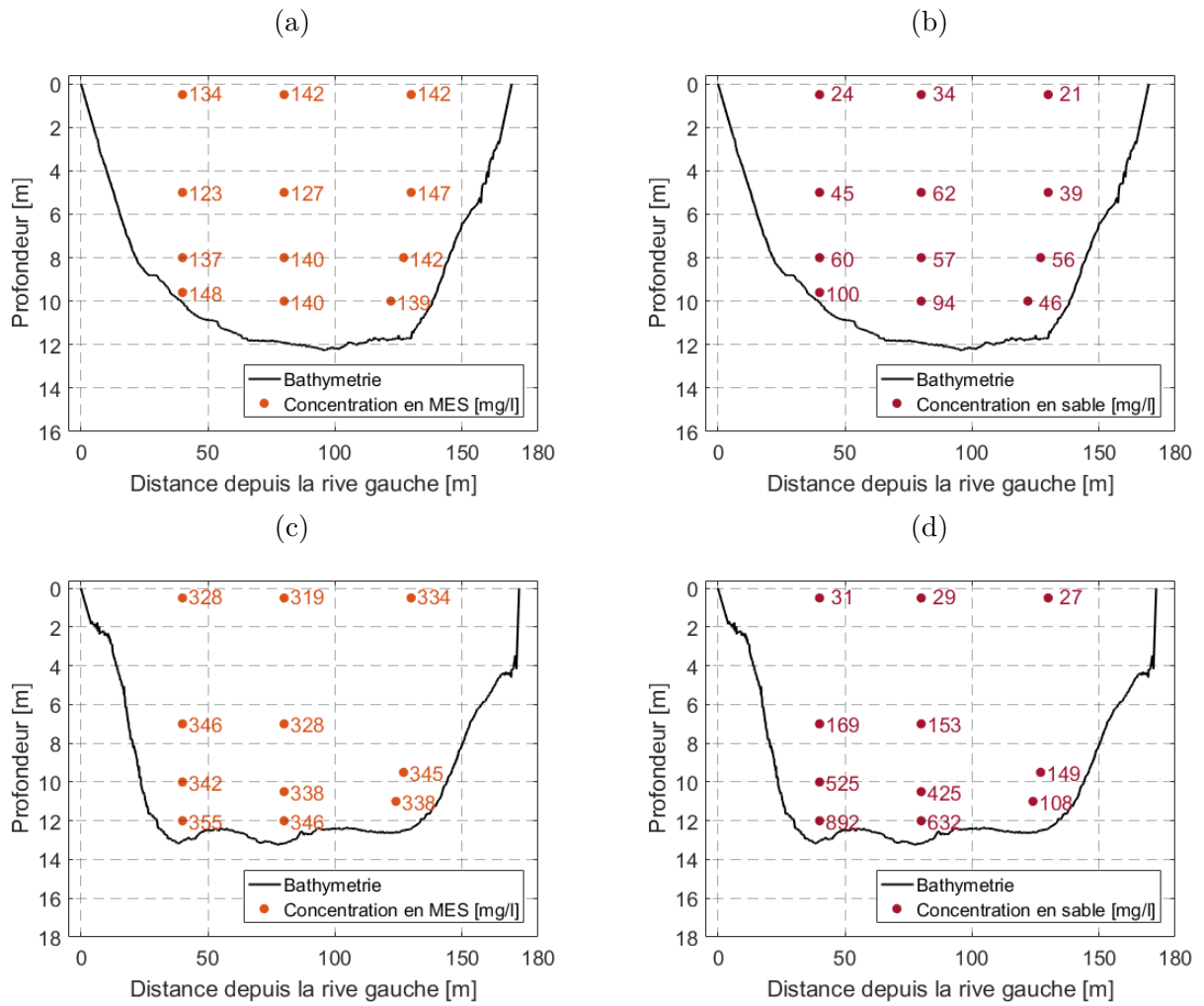
FIGURE 2.21. Répartition des concentrations dans la section sur le Rhône à Perrache les 22 et 23 janvier 2018 : concentrations en fines avec séparation des sable (a et c) et concentrations en sable après séparation (b et d).
