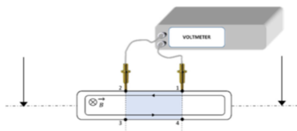
Fig. 1- Schéma descriptif de la méthode des pointes magnétiques
