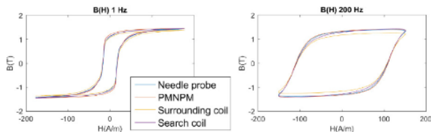
Fig.4 Comparaisons cycle d'hystérésis, 1 – 200 Hz.
