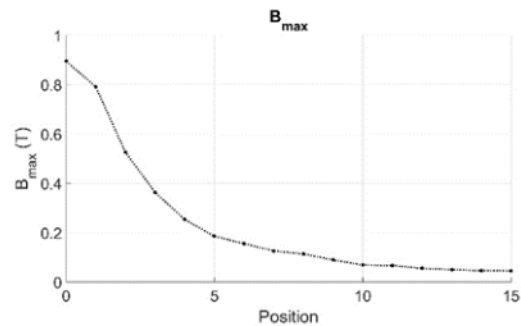
Fig. 6 - Champ induit maximal en fonction de la position de la tôle instrumentée
