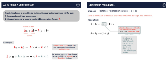
Fig. 1. Exemples de rétroactions. Type < J ; G ; C ; null > et < P ; I ; C ; Er_oublCofacteur1 >
