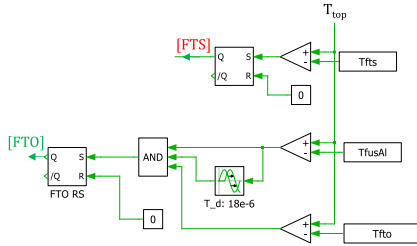
Fig 14. Blocs de comparaison pour l'activation des modes de défaillance FTO et FTS par la température simulée sur la ligne de Cauer n°2 : T_{fts\ corrected} = 2400K , T_{fuseAl} = 933K , T_{fto\ corrected} = 1900K .
