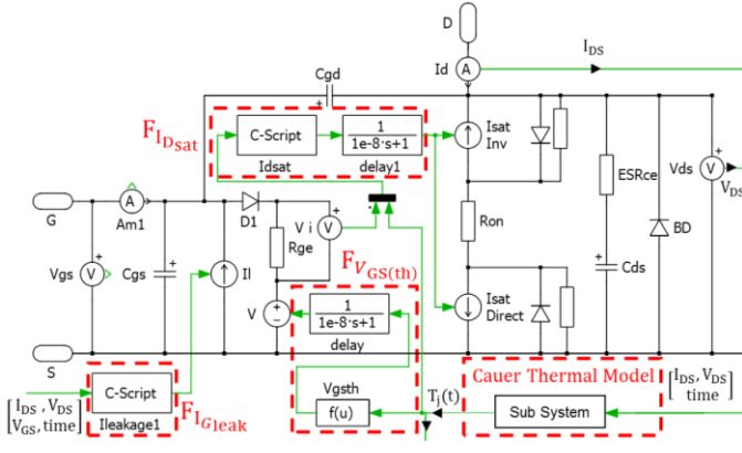
Fig. 11. Modèle électro-thermique compact du Mosfet SiC pour des besoins de représentation en mode de court-circuit : FI_{Dsat} , FI_{Dsat} représentent respectivement les fonctions de comportement I_{Gleak}(T_j) , V_{GSth}(T_j) and I_{Dsat}(T_j) .
