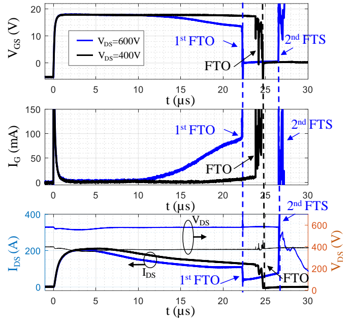
Fig. 8 Formes d'ondes expérimentales d'un Mosfet SiC 1,2kV – 80mΩ à grille planar en court-circuit sous V_{buffer(on/off)} = 18V/-5V , R_{Gate Ext.} = 47\Omega , T_{jinit} = 25^\circ C : courbes en noir V_{DS} = 400V , courbes en bleu V_{DS} = 600V . Cas d'un pulse de court-circuit dit "long" sans blocage par la commande.
