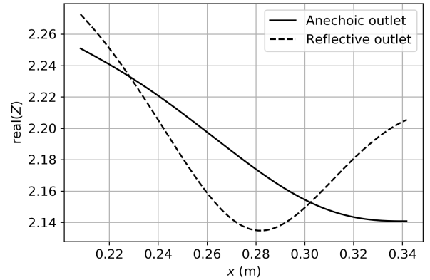
(d) Converged impedances. Z_{\text{ref}} = 2
