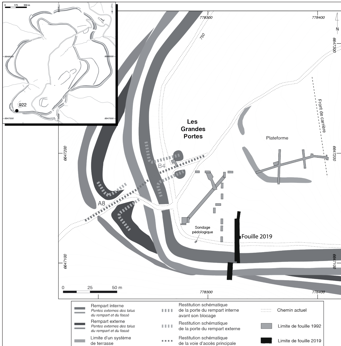
Fig.1 : Localisation de la fouille 2019 et restitution schématique des fortifications des Grandes Portes (DAO Bibracte/A. Meunier)
