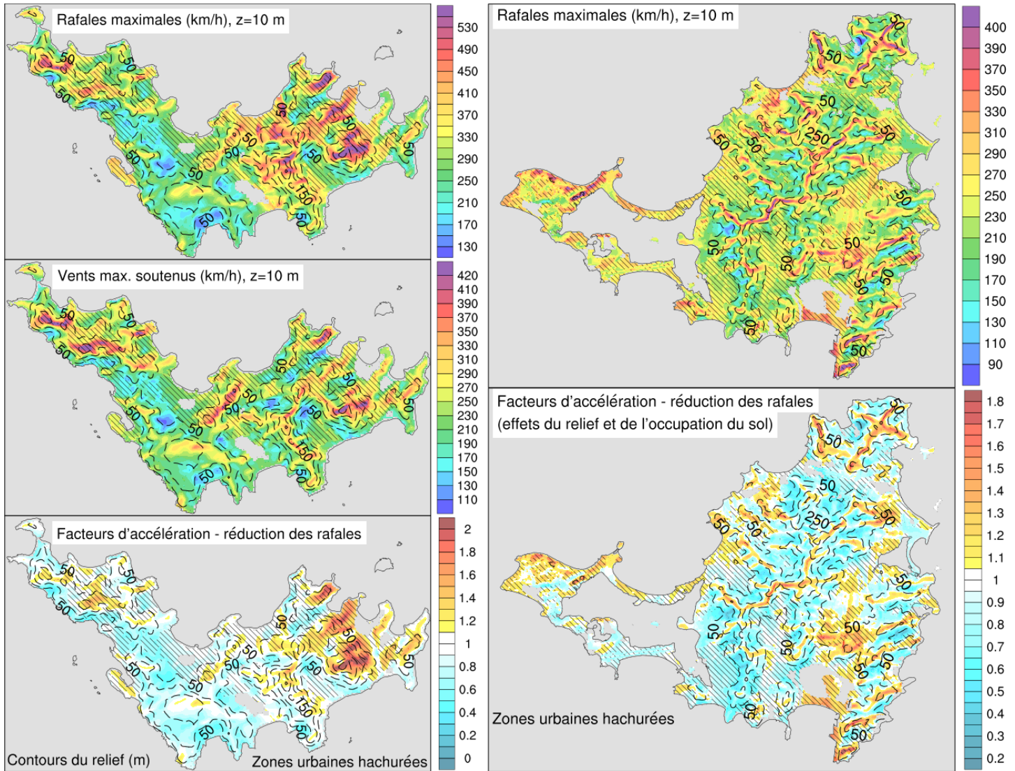
Simulations WRF à 30m de résolution : rafales max. (km/h), vents max. soutenus 1 min (km/h), facteurs d'accélération - réduction des rafales : Saint-Barthélemy (colonne gauche) et Saint-Martin (colonne droite) (Cécé et al. 2020)
