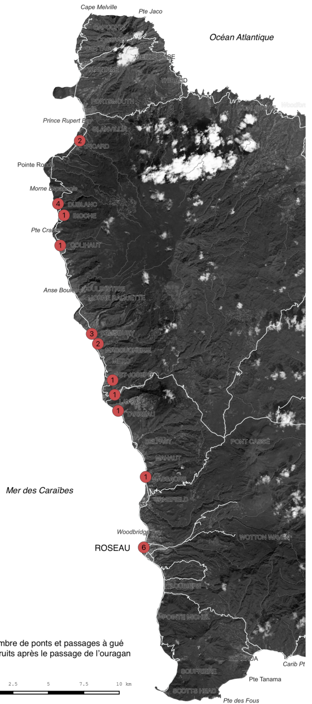
Recensement des dommages aux ponts et passages à gués suite au passage de l'ouragan Maria sur la côte occidentale de la Dominique (Battut, 2019).
