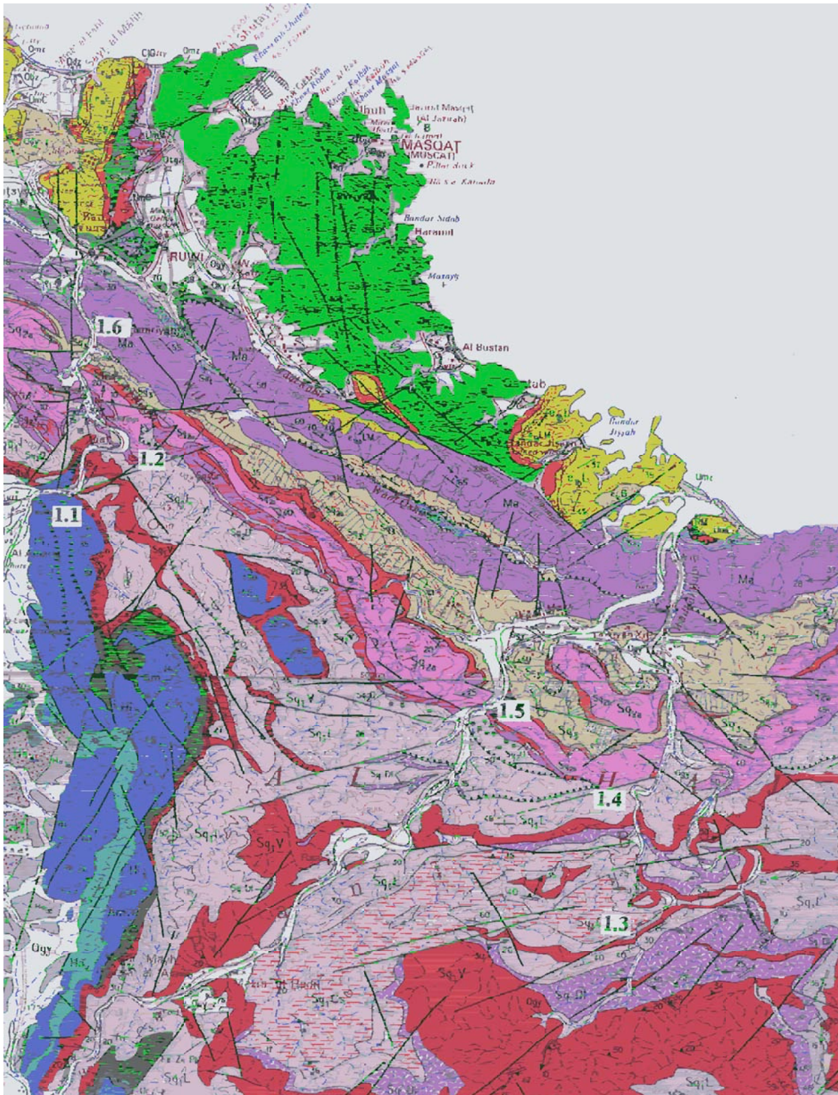
Figure 7– Geological map of the Wadi Aday – Wadi Mayh – Wadi al Hulw area, Saih Hatat region (Scale 1:100 000 ; Le Métour et al. 1986 a&b)
