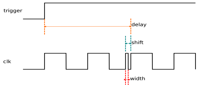
Fig. 2. Clock glitch parameters
