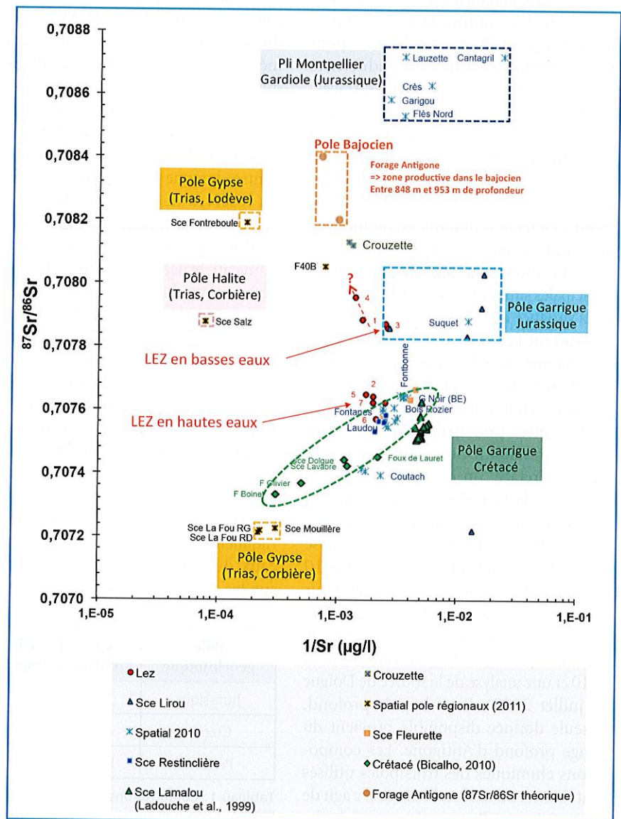
Figure 4: Rapport 87 Sr/ 86 Sr des eaux du système karstique du Lez et des systèmes karstiques environnants en fonction du rapport (1/Sr). Les pôles géochimiques régionaux sont également reportés. 87 Sr/ 86 Sr ratio for the Lez karstic spring waters and for the surrounding karst systems versus 1/Sr ratio. Regional geochemical end-members are plotted on.
